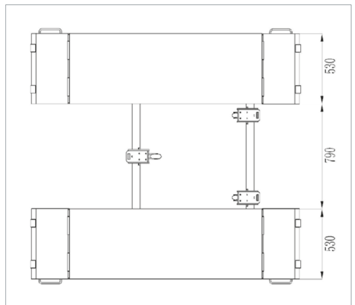
Pulverbeschichtete Ausführung ATH-Flex Lift 30 Artikelnummer: 680008
