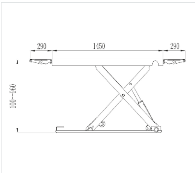
Feuerverzinkte Ausführung ATH-Flex Lift 30Z Artikelnummer: 680008-FZ
