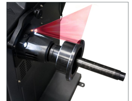
Gewindewelle (mit Laser und Licht) Thread shaft (with laser and light) Axe fileté (avec laser et lampe)
